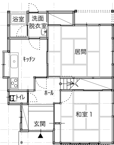
改修前 1階 平面図
