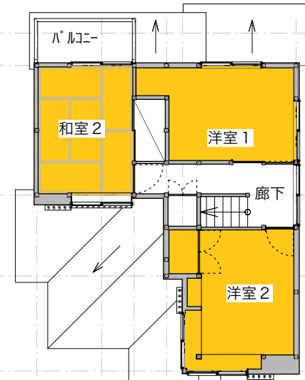
改修後 2階 平面図
