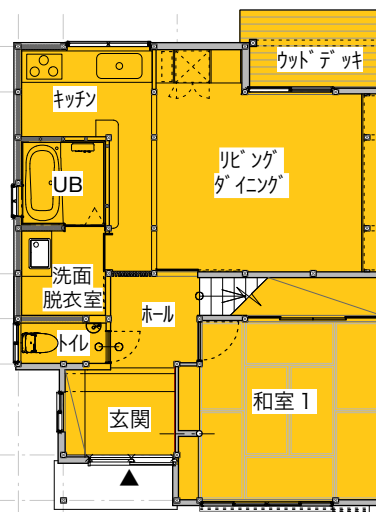
改修後 1階 平面図
